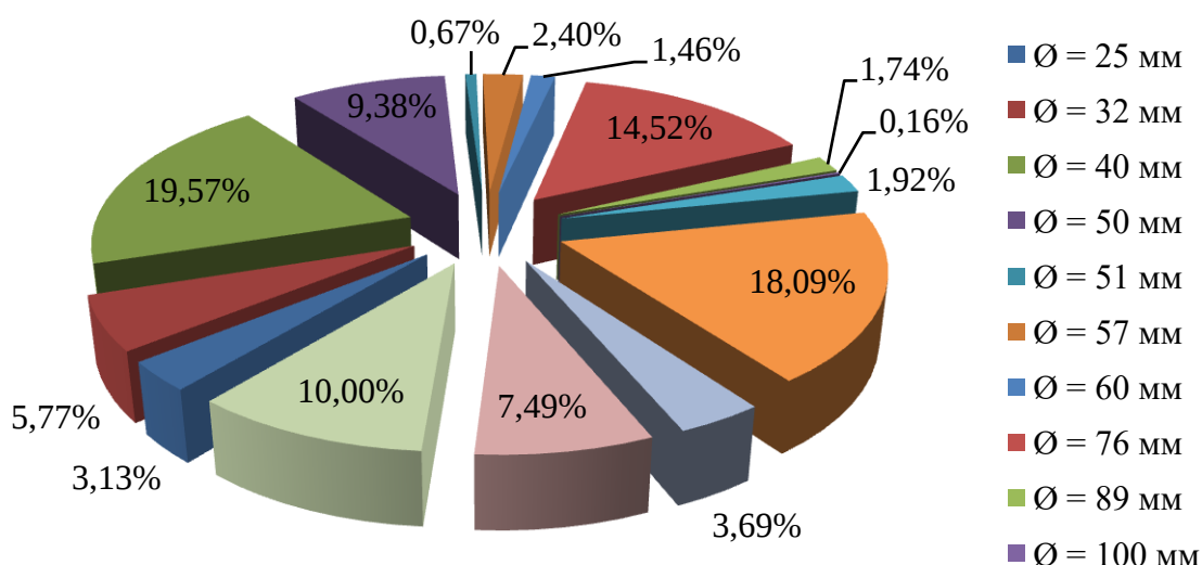
Рисунок 2.3.2.2 – Доли протяжённости участков трубопроводов тепловых сетей котельных МУП «Энергетик» различных диаметров
