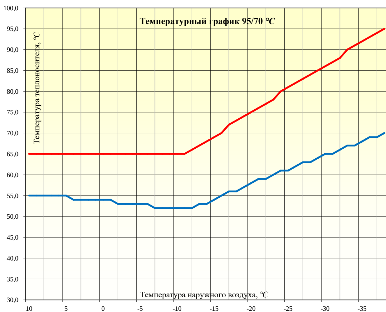
Рисунок 2.3.5.2 – График регулирования отпуска тепла тепловые сети от котельной, № 2, с. Лесное – 95/70 °C
